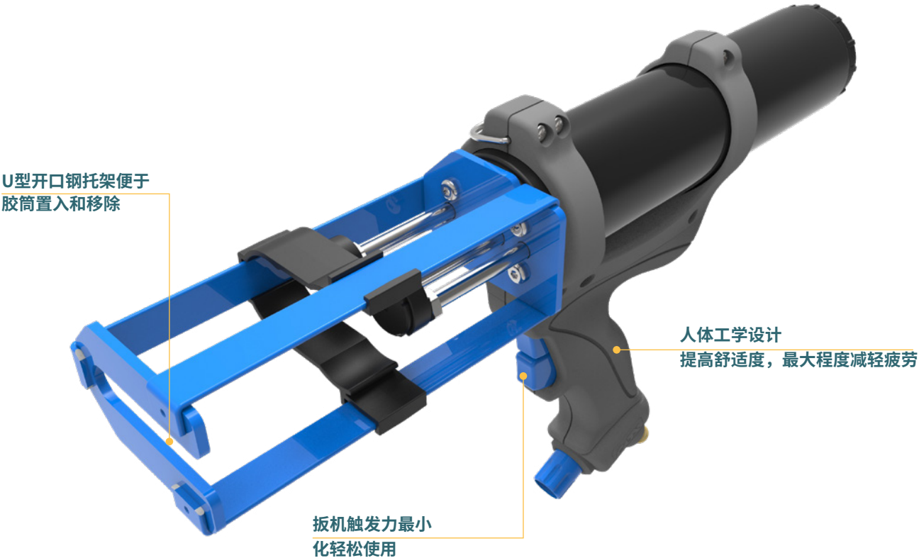
展示型号: AirFlow 3 VBA 200B MR 200 mL
