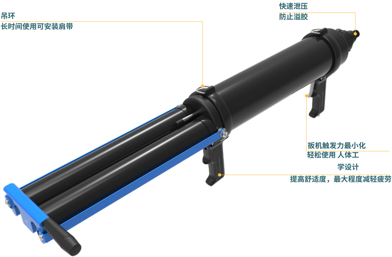
展示型号: AirFlow 1 CBA 600S 1200 mL
