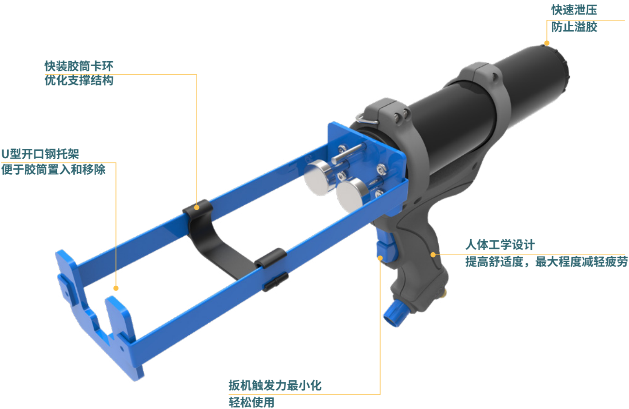
展示型号: AirFlow 3 VBA 100 HP 200 mL
